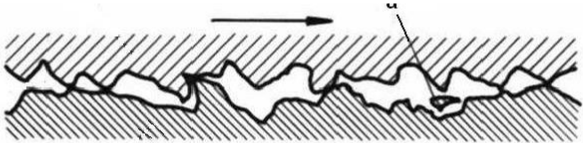
Figuur 1: Bij stilstand van de glijlagers is er metaal op metaal contact. Door de grote wrijving ( \mu groter dan 0,3) is er ook sprake van grote slijtage. Stukjes metaal kunnen afbreken (a).
