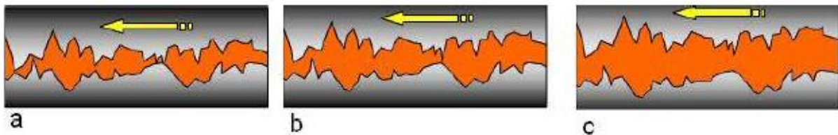
Figuur 2: a) grenssmering, de metaaltoppen raken elkaar constant. b) gemengde smering, de metaaltoppen raken elkaar licht. c) volkomen smering, de oliefilm scheidt de metaaldelen volledig
